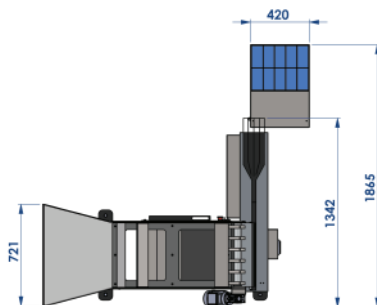
Dimensões básicas.
